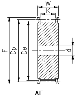
T5型标准皮带宽 (25mm)
