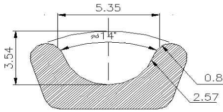
8M型齿形图:
