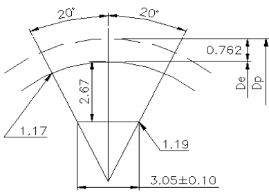
L型齿形图:
