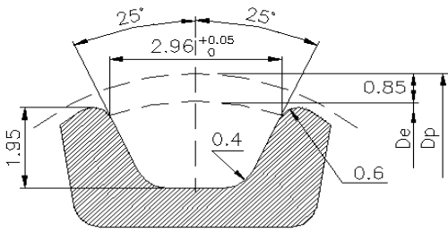
T5型齿形图:
