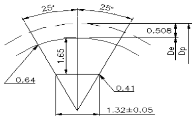
XL型齿形图:
